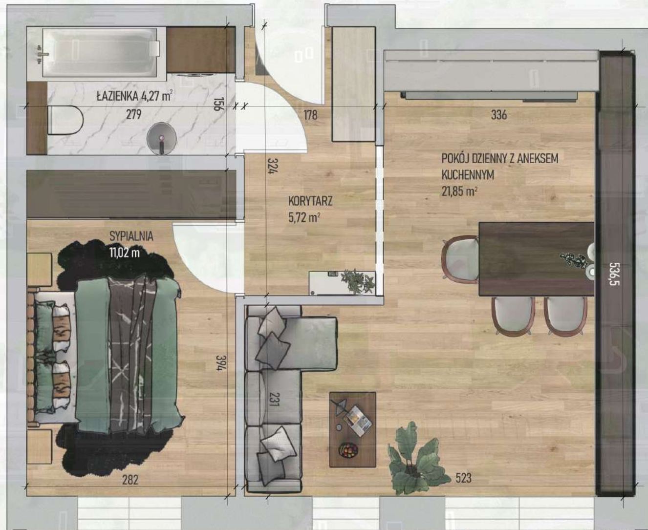
RZUT MIESZKANIA NR 1/ M37
