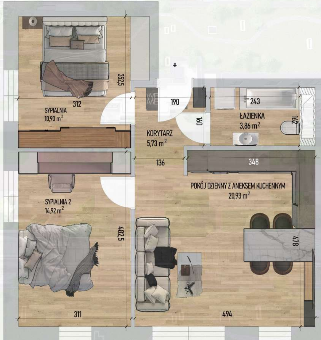
RZUT MIESZKANIA NR 1/M6
