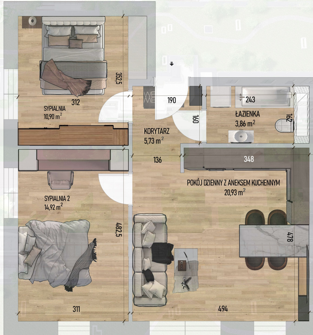
RZUT MIESZKANIA NR 1/ M21
