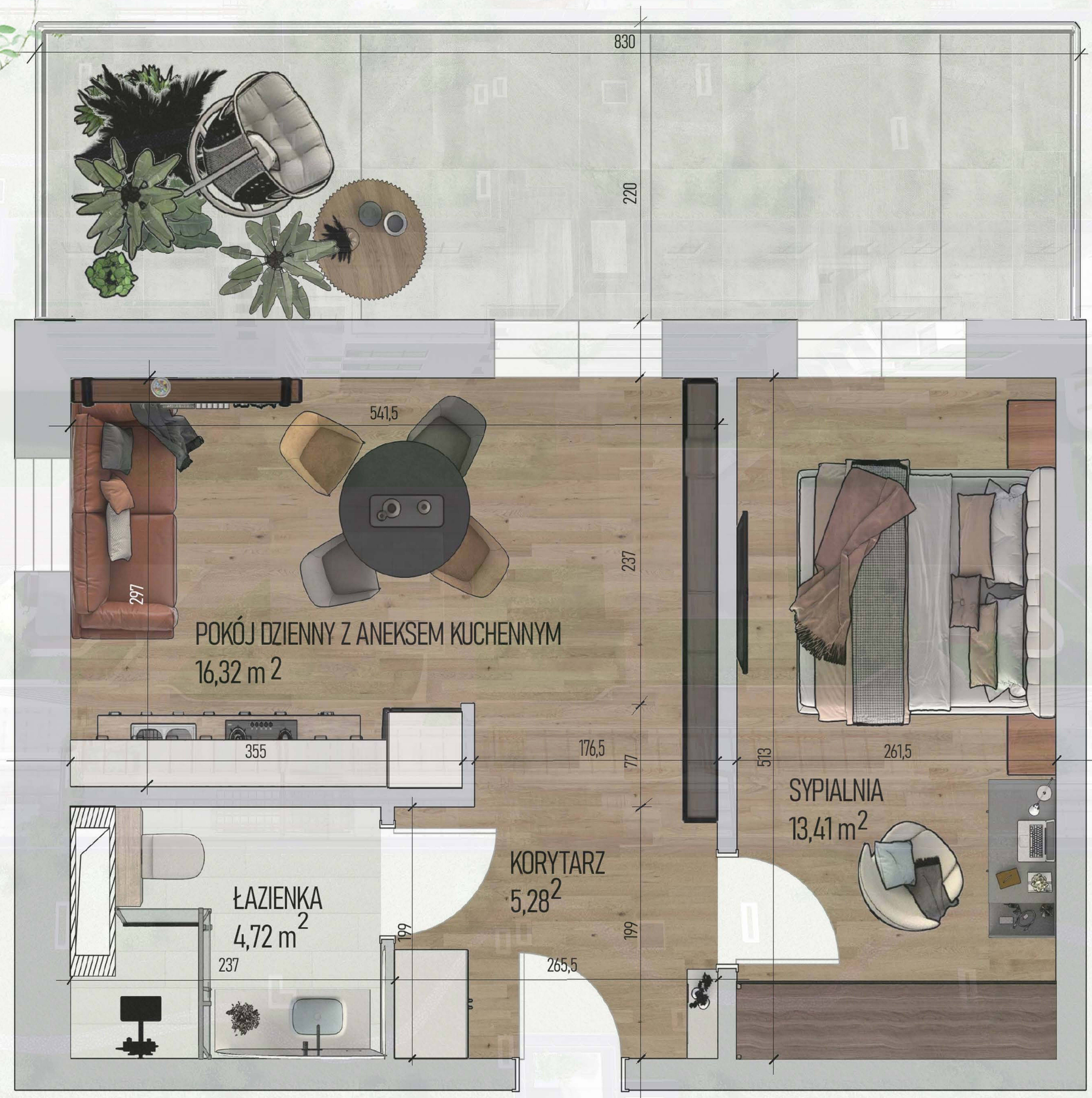
RZUT MIESZKANIA NR 1/ M1
